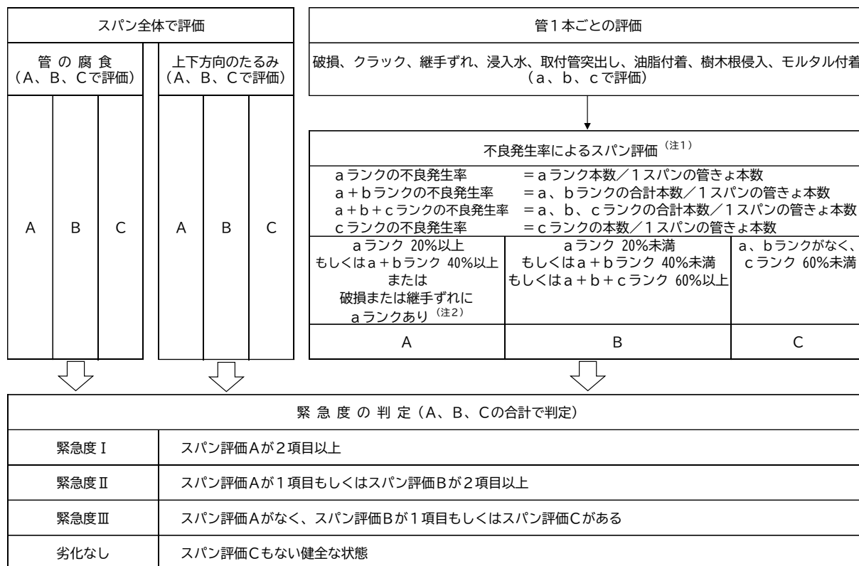
図－２－１ 緊急度の判定基準【鉄筋コンクリート管等(遠心力鉄筋コンクリート管含む)及び陶管】
